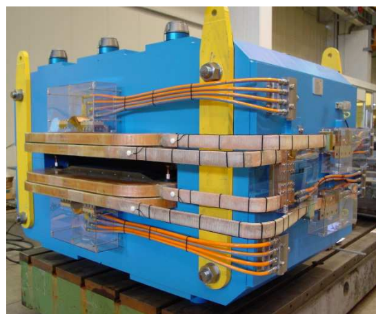
HEBT switching dipole
