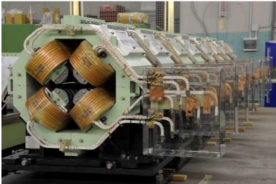
HEBT quadrupole magnet
