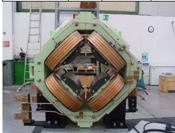
Quadrupole magnet
