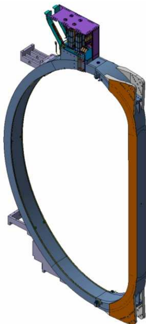
TF coil: overall dimensions 8,3 x 4,5 x 0,6 m weight 15,5 t
